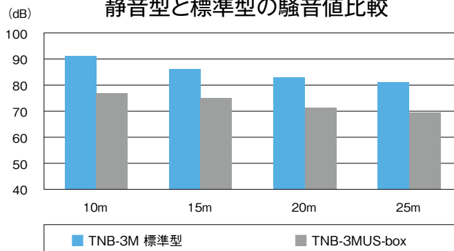
静音型と標準型の騒音値比較
