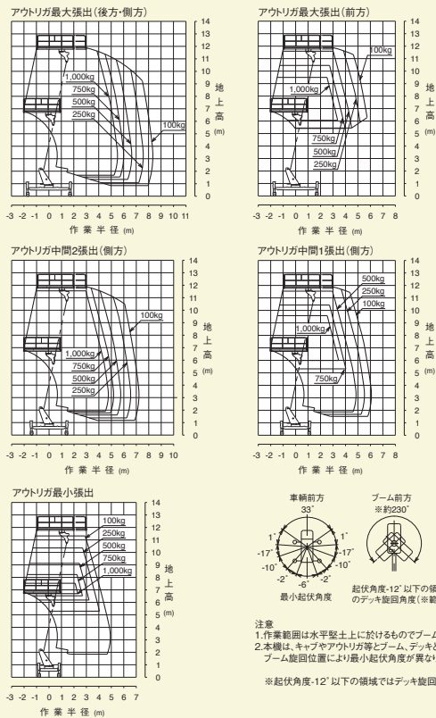
作業範囲図
