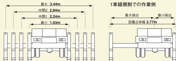
アウトリガ
