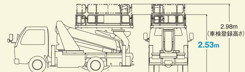
手すり展開時
