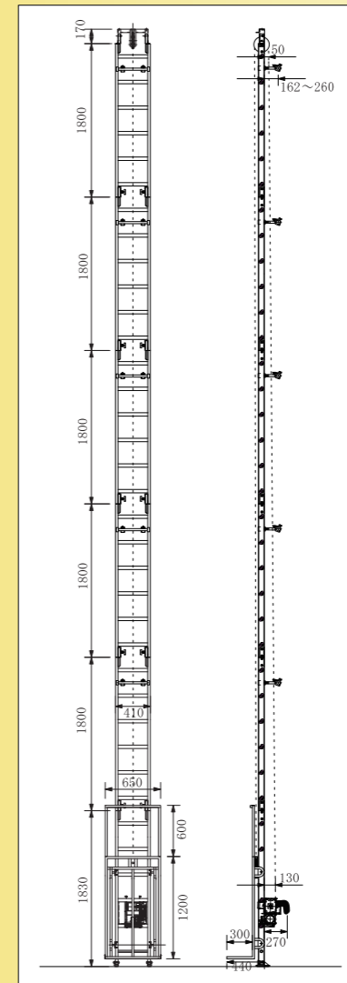
■図面 (mm)
